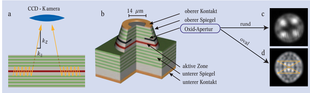
Schematischer Strahlengang (a) und lithographische Struktur (b) eines VCSELs. Gegenläufige Wellenzüge, die vom seitlichen Rand reflektiert werden, überlagern sich zu stehenden Wellen im transversalen Profil. Diese Intensitätsverteilung wird durch die Öffnung im oberen Kontakt emittiert und von einer
